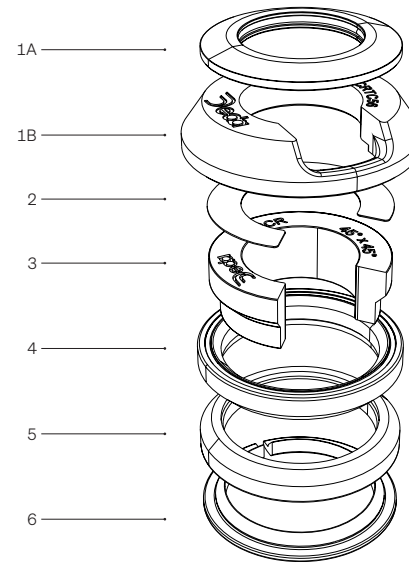
Esploso S-DCR Spare parts S-DCR
