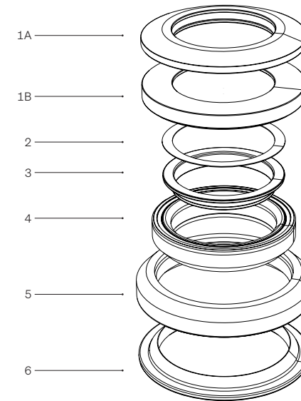
Esploso IN5 / IN4 Spare parts IN5 / IN4
